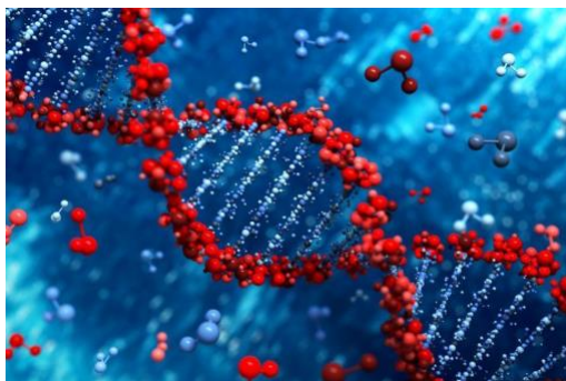
Molekula DNK
